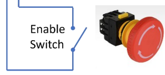
스위치 회로의 전류 : 100mA 이하. 비상스위치를 달아서 사용하면 좋음
